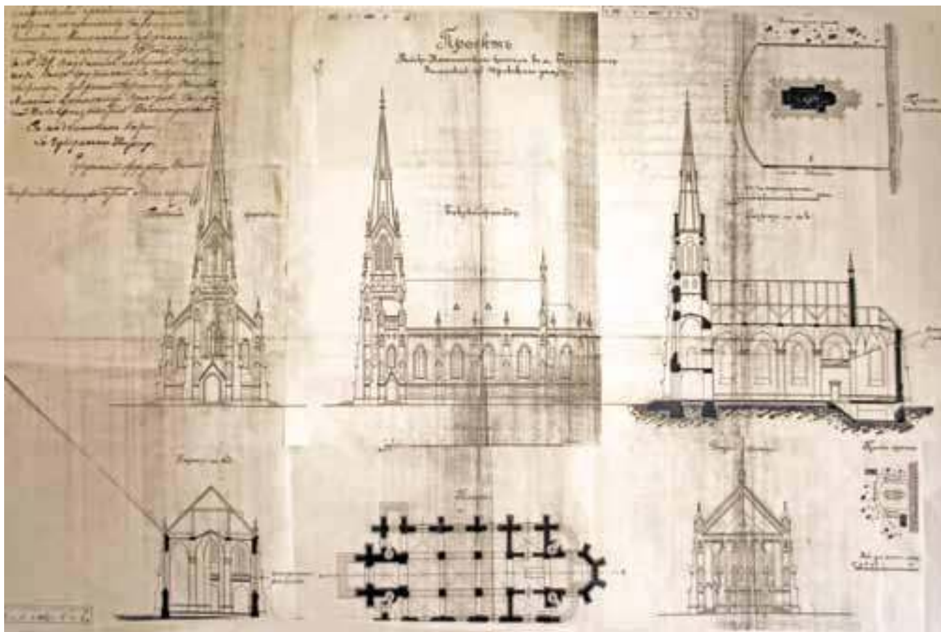
Bendras archyvinis bažnyčios projektas (LVIA)
